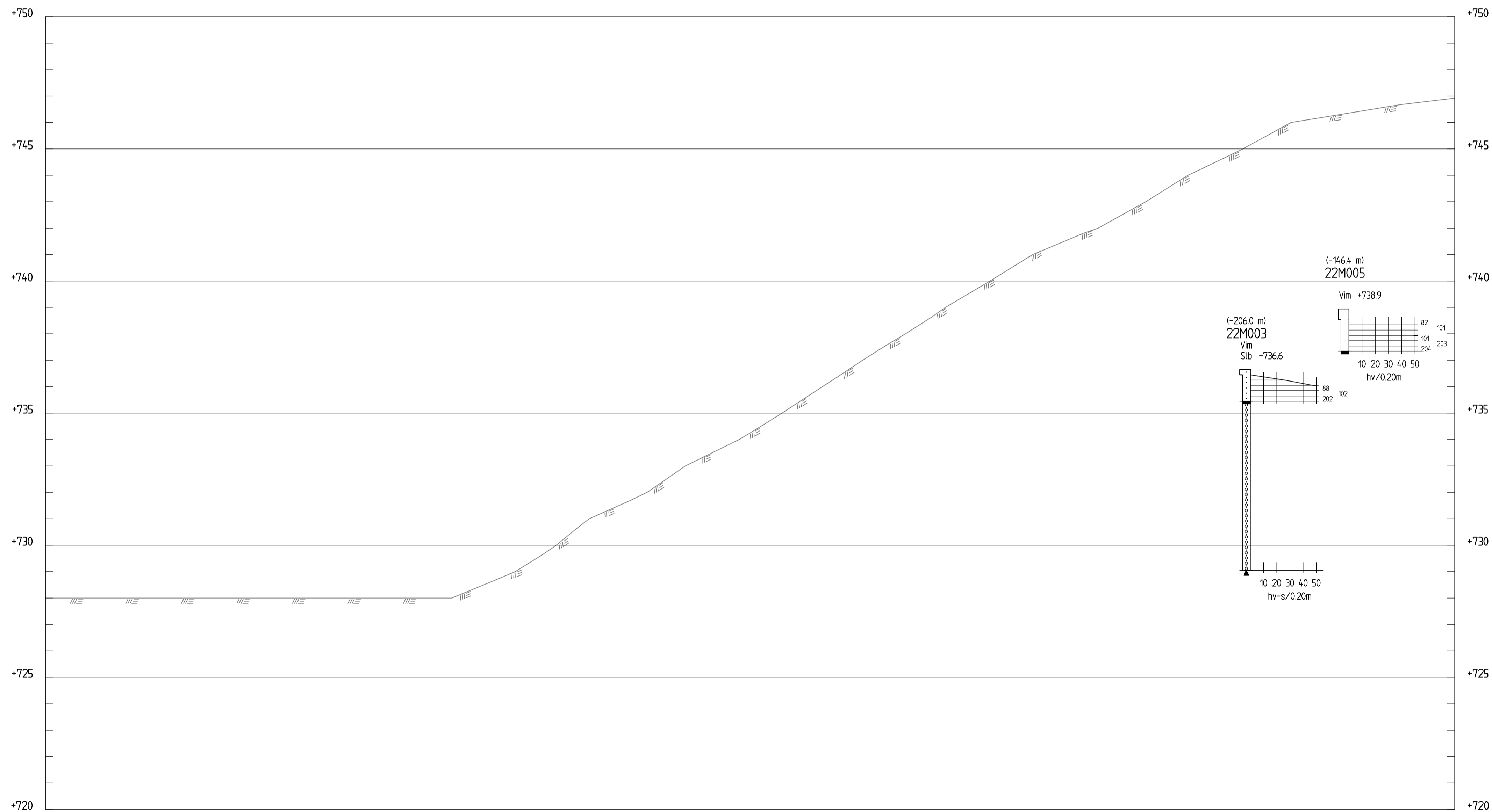
SEKTION F-F 1:100
